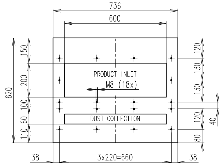
TOP FLANGE
