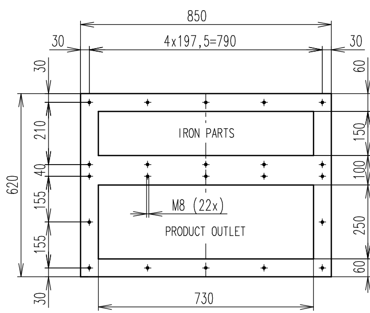
BOTTOM FLANGE
