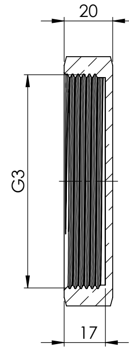
SCHNITT A-A
